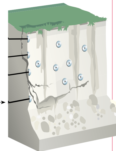
Principe de la parade par ancrage du rocher
