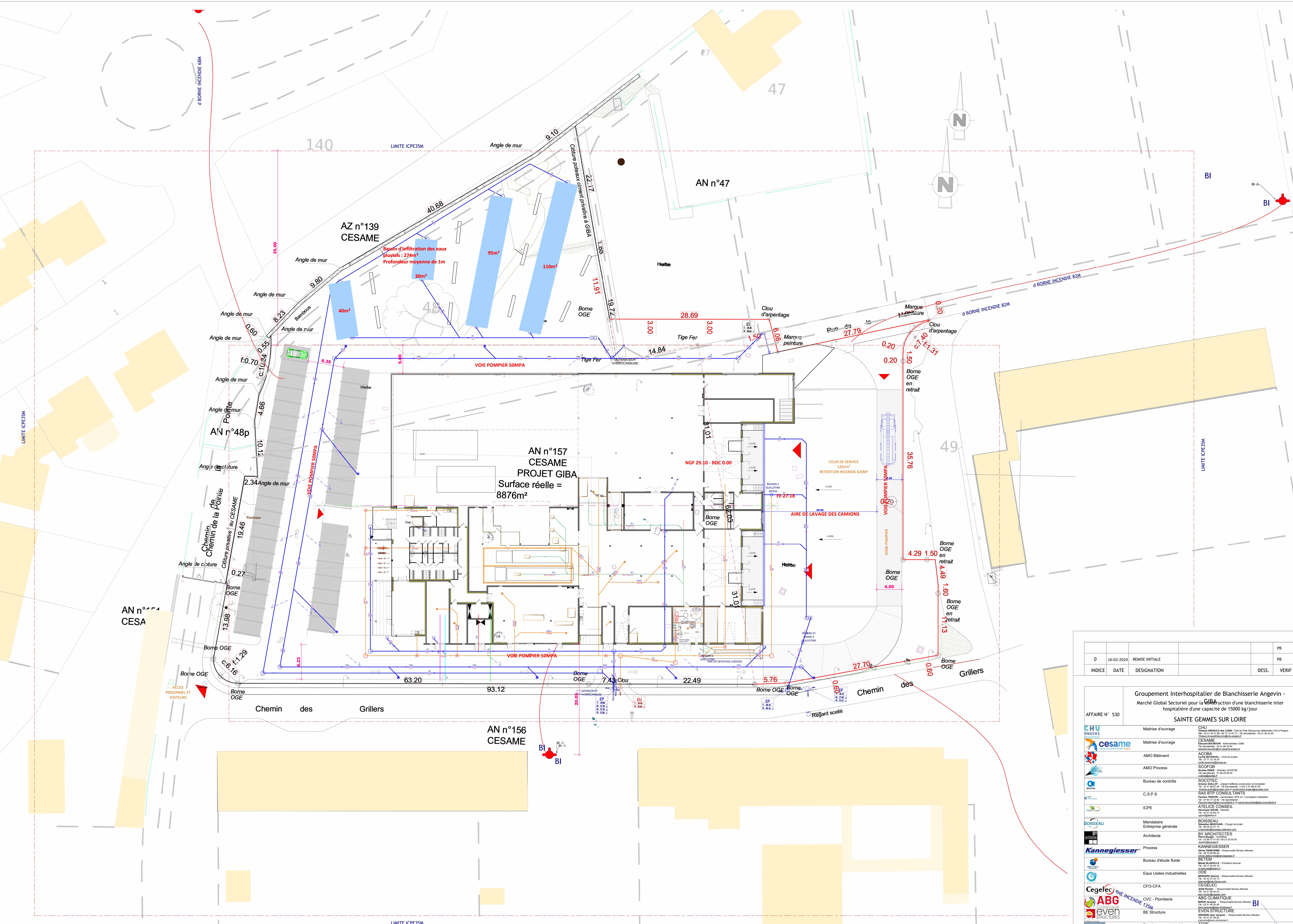
PLAN RESEAUX SUR RDC 1 : 200
